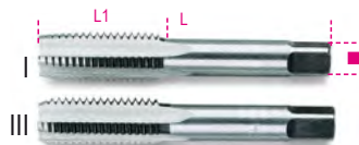
DIN 2181 UNI 4535
