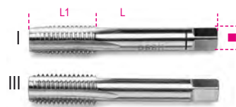
DIN 2181 UNI 4535
