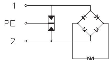
Kapcsolási rajz
