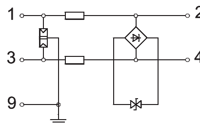
Kapcsolási rajz
