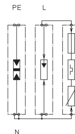
Kapcsolási rajz
