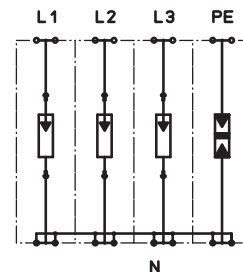
Kapcsolási rajz
