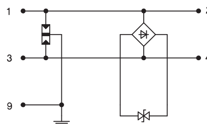
Kapcsolási rajz
